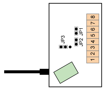
Funkmodul mit Jumper JP1-JP2-JP3
